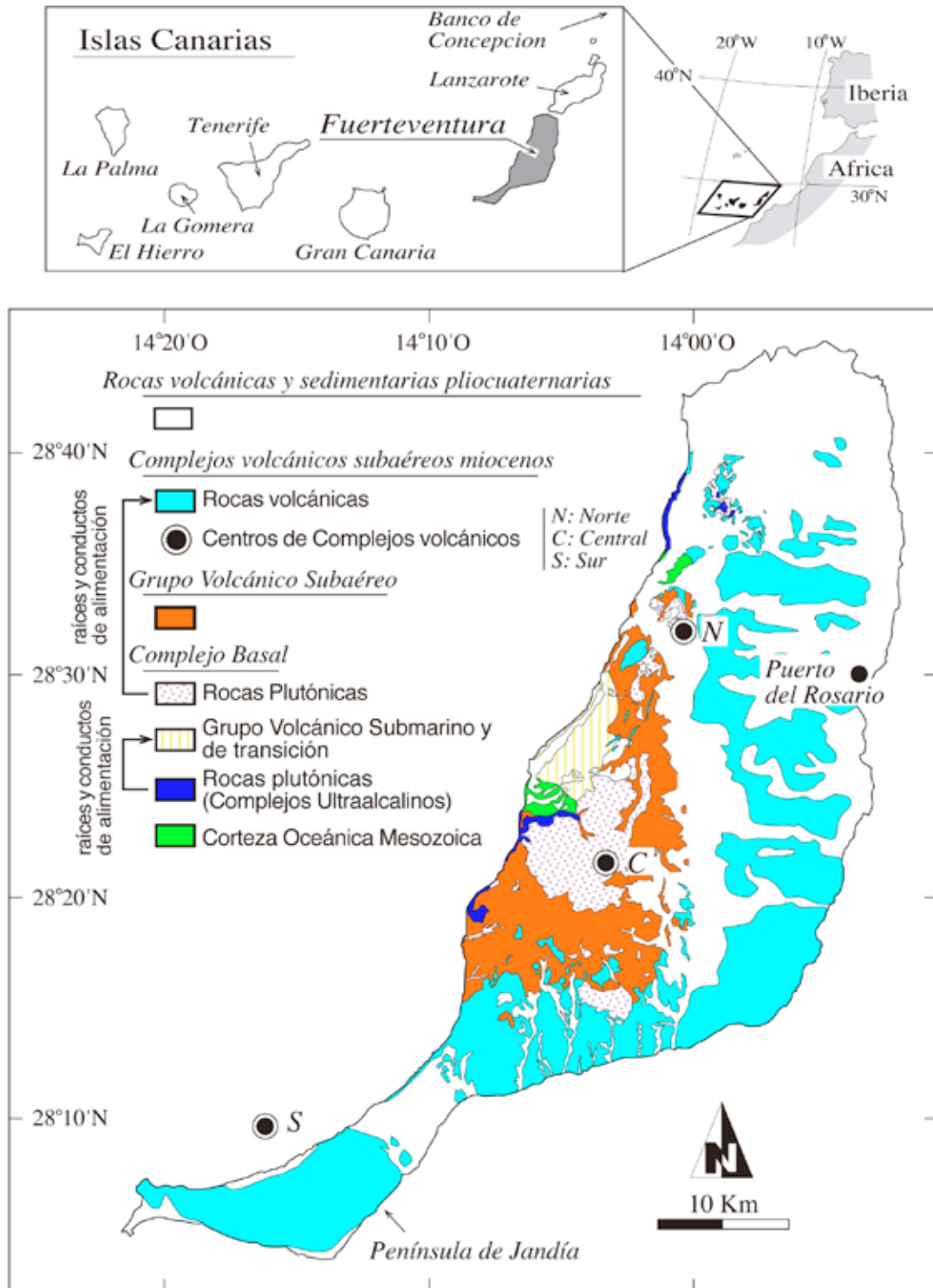
Fig. 2.- Esquema geológico de la Isla de Fuerteventura mostrando las principales unidades, la localización de los centros de los edificios volcánicos miocenos (N: Norte, C: Central, S: Sur). El principal afloramiento del Complejo Basal, en la zona centro-occidental de la isla, es el llamado Macizo de Betancuria (tomado de Casillas et al., 2008).
